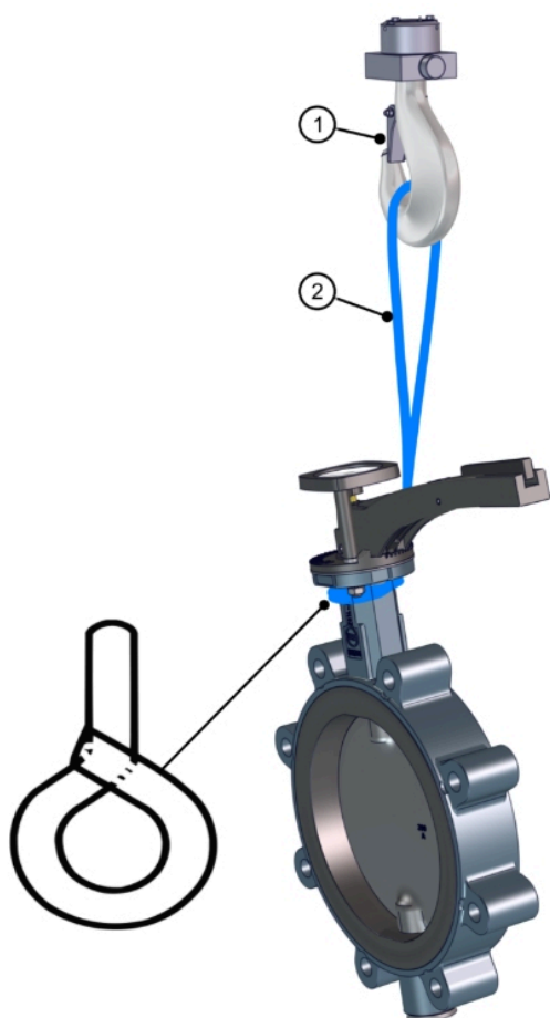
Obr. 6: Přepravte klapku příruby jeřábem
