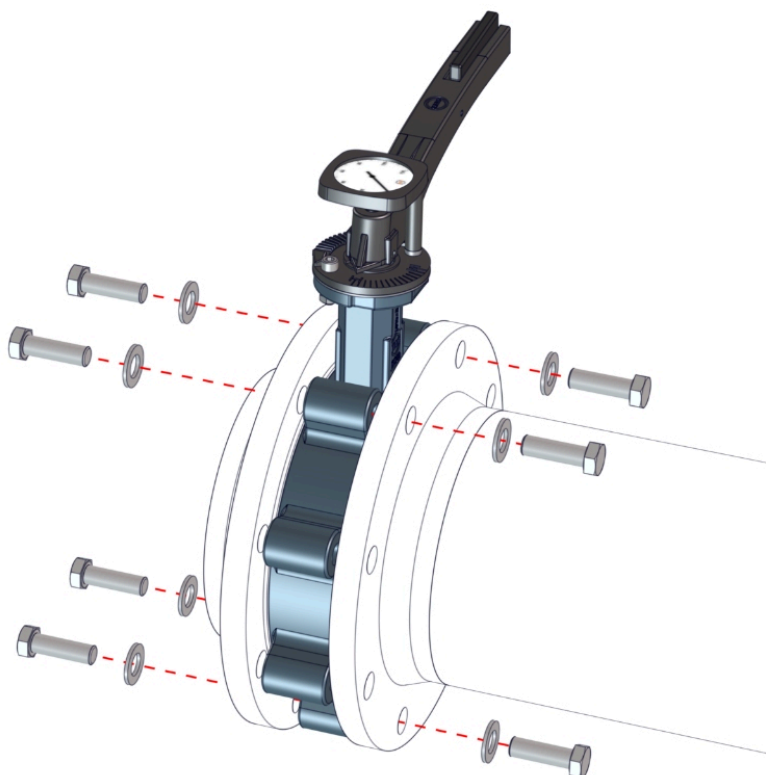
Obr. 8: Polohování klapky příruby
