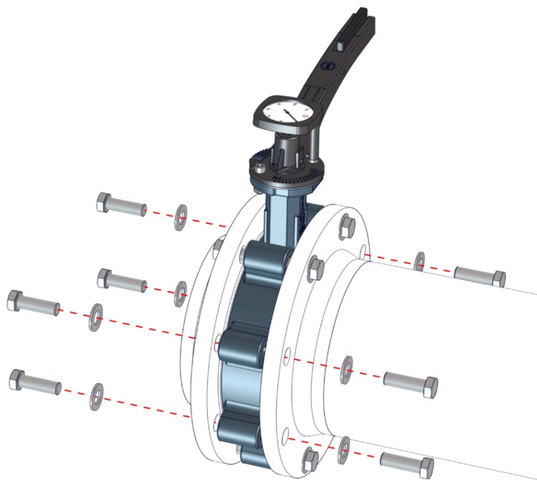
Obr. 9: Přišroubování klapky příruby
