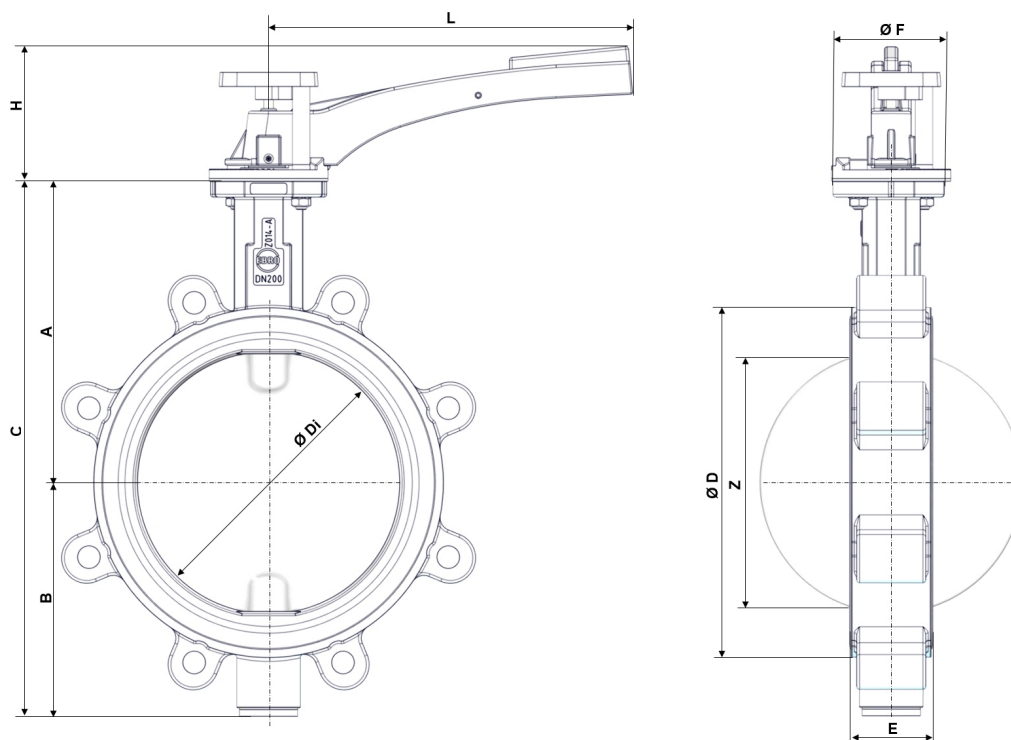
Obr. 3: Hlavní rozměry Z014-A THERM
