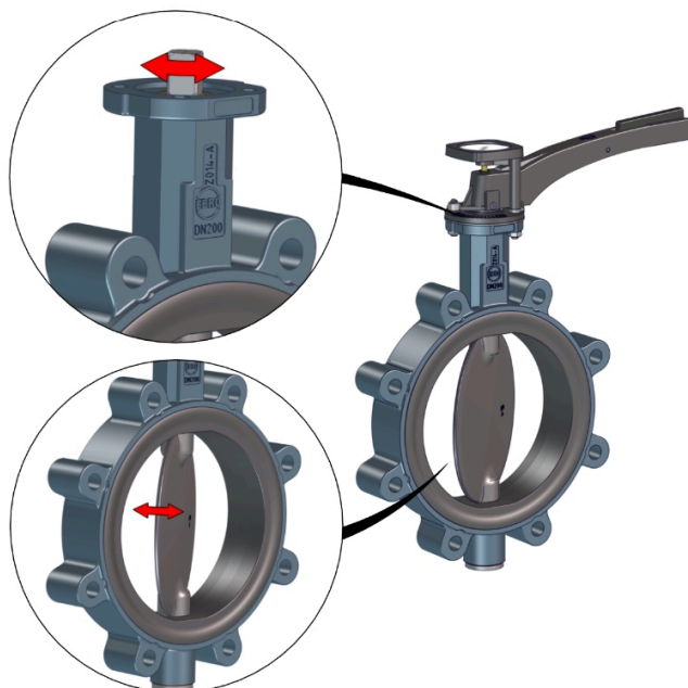
Obr. 4: Pohyblivé díly
