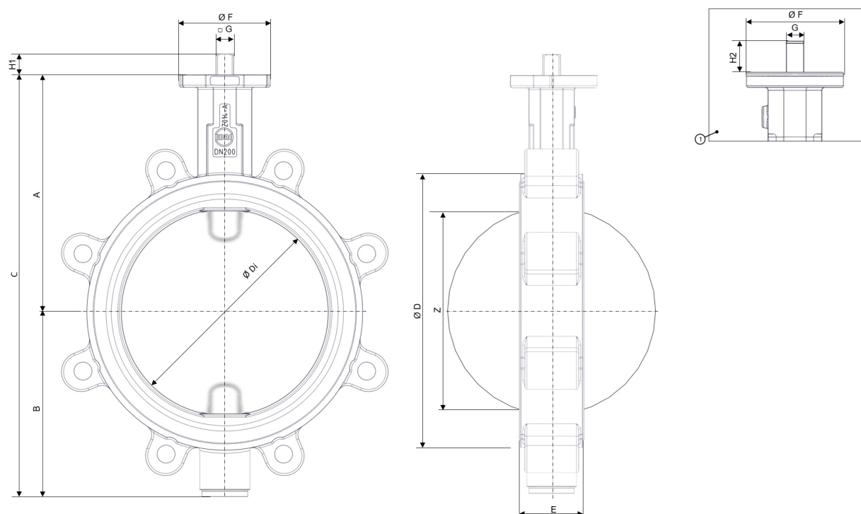
Obr. 3: Hlavní rozměry Z14-A
