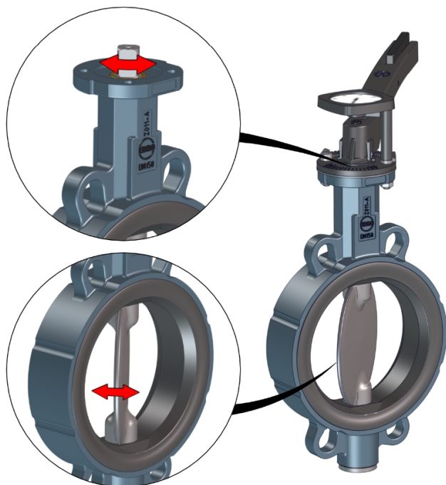
Obr. 4: Pohyblivé díly
