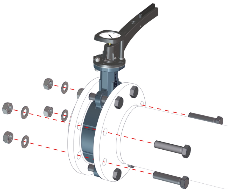
Obr. 9: Přišroubovat klapku vložené příruby
