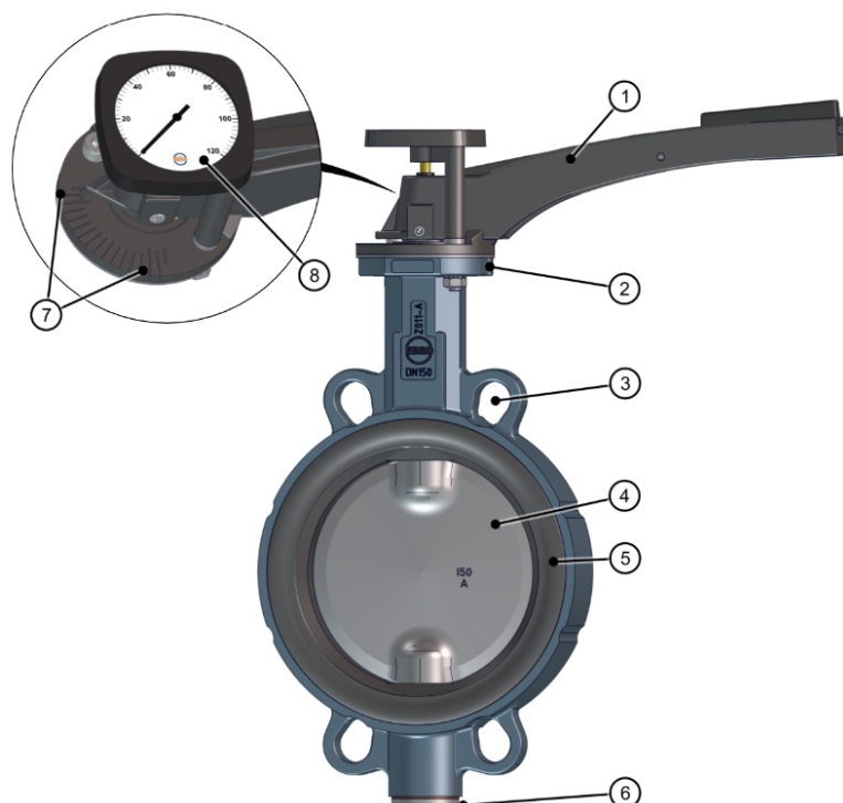
Obr. 2: Komponenty
