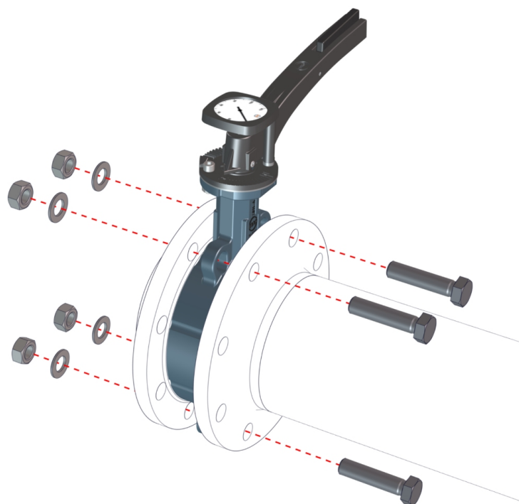
Obr. 8: Polohovat klapku vložené příruby
