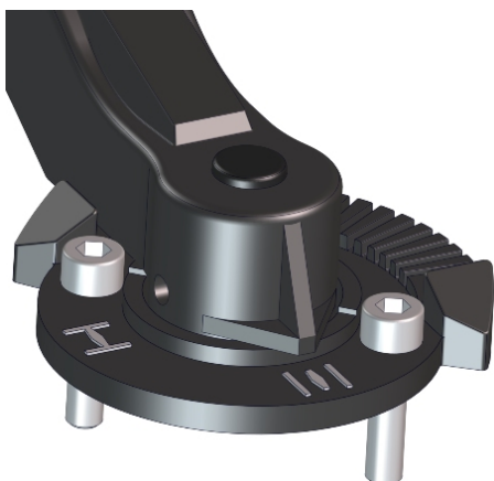
Obr. 15: Indikátor polohy
