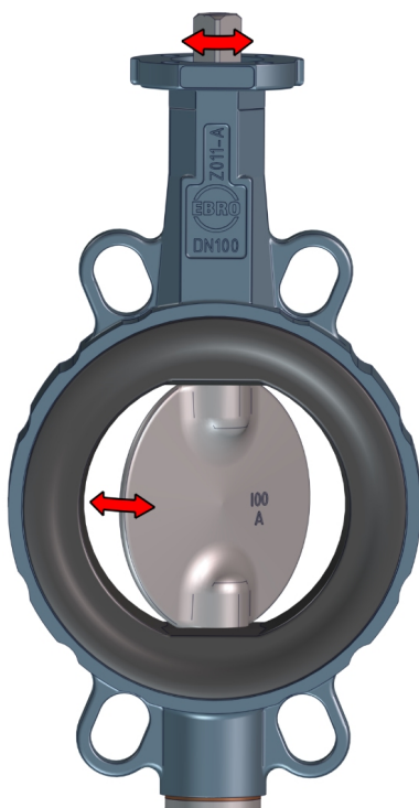
Obr. 4: Pohyblivé díly
