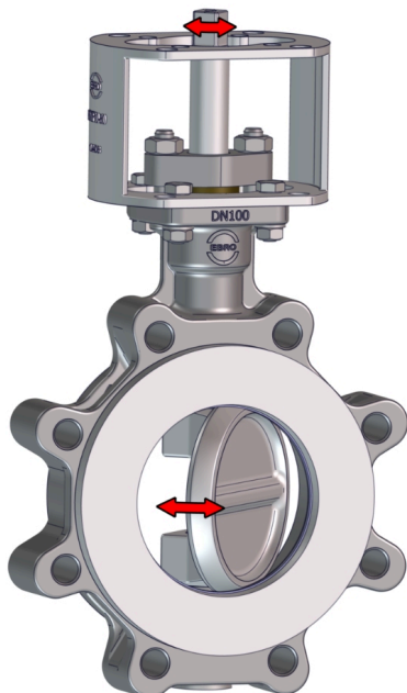
Sl. 4: Pokretni dijelovi
