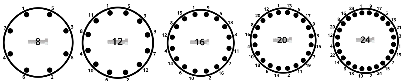
Sl. 12: Redoslijed navojnih spojeva priрубnice za cijev
