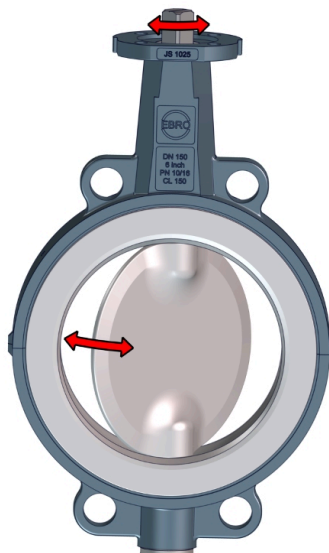
Sl. 4: Pokretni dijelovi
