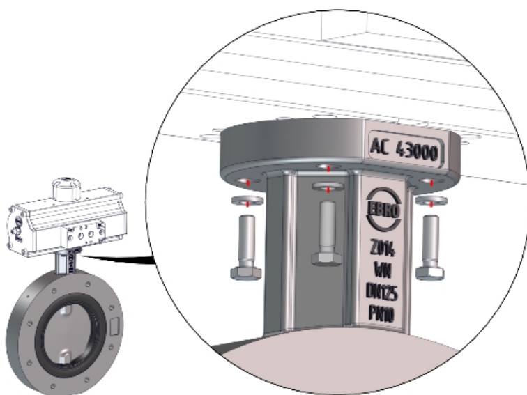
Sl. 7: Princip za montiranje komponenti
