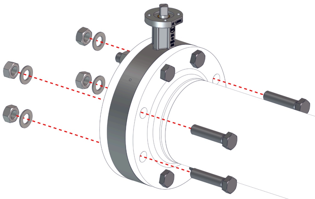
Sl. 9: Zavijčati klapu pune prirubnice
