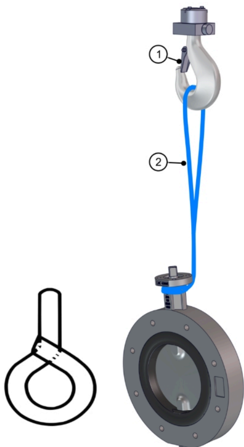
Sl. 6: Klapu pune priрубnice postaviti na kran
