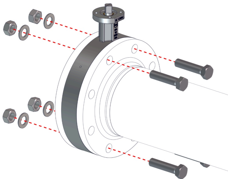
Sl. 8: Pozicionirati klapu pune prirubnice
