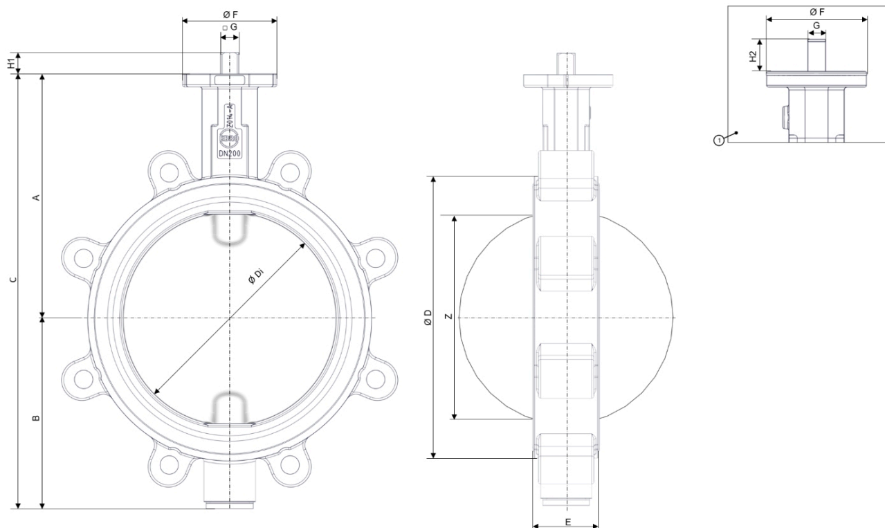
Sl. 3: Glavne dimenzije Z014-B
