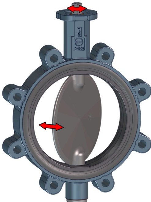
Sl. 4: Pokretni dijelovi
