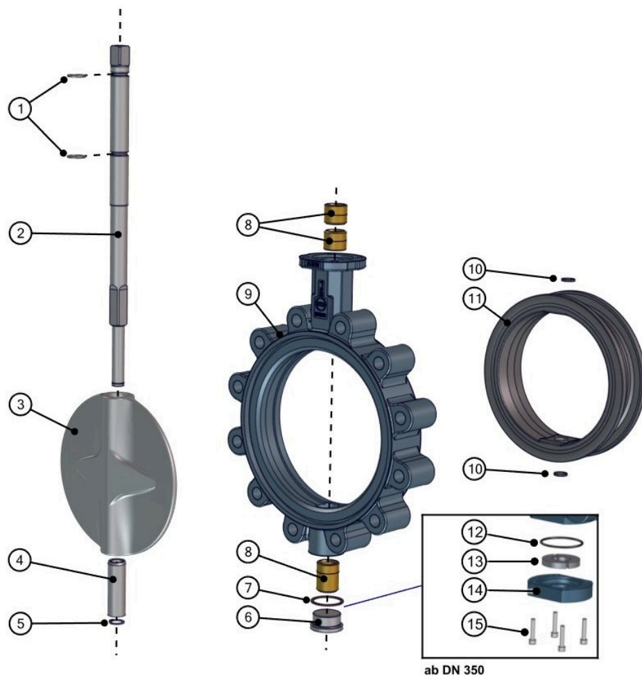
Sl. 16: Sastavnica Z014-A TS-vratilo
