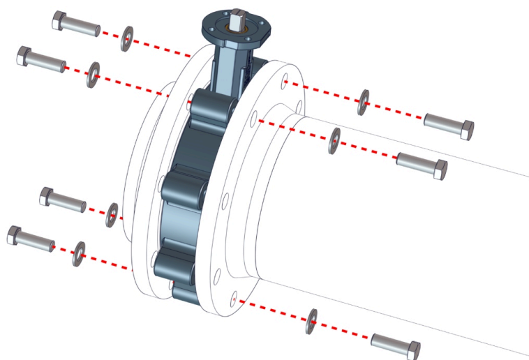
Sl. 8: Pozicionirati klapu prirubnice
