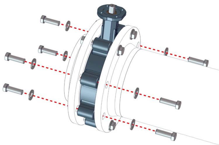
Sl. 9: Zavijčati klapu prirubnice
