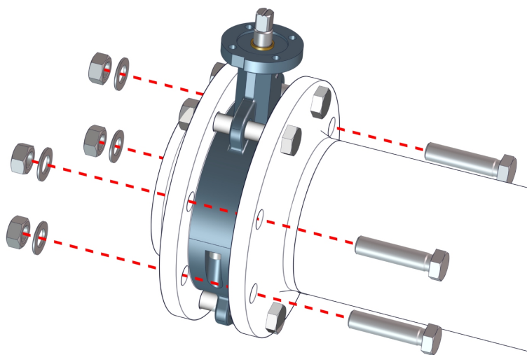
Sl. 9: Zavijčati klapu međuprirubnice
