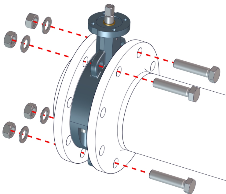
Sl. 8: Pozicionirati klapu međuprirubnice
