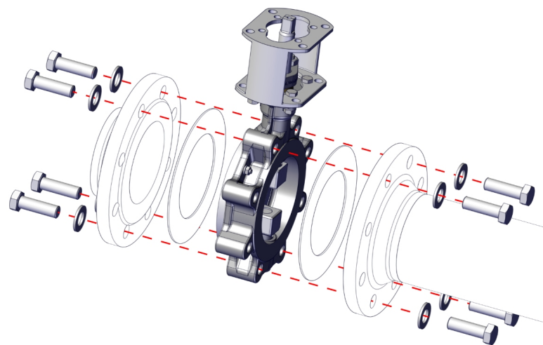
图 8: 定位法兰连接罩
