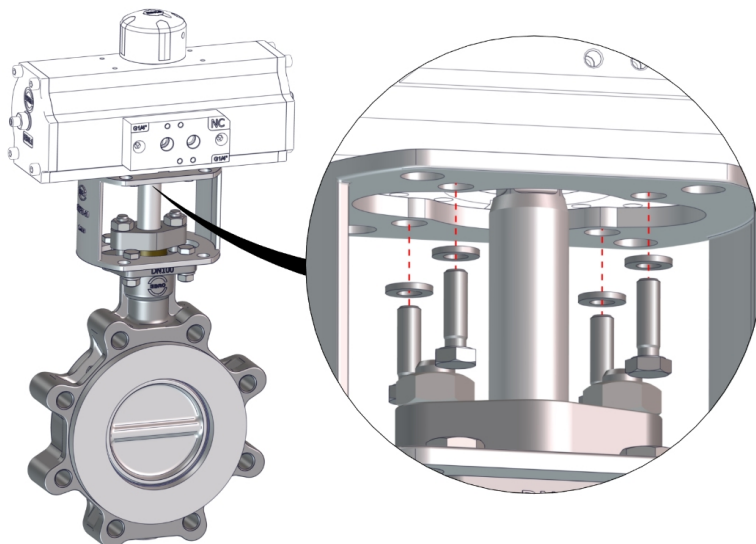
图 7: 安装组件的原理
