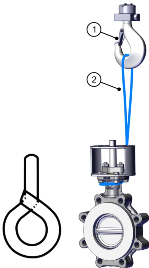
图 6: 起吊法兰连接罩
