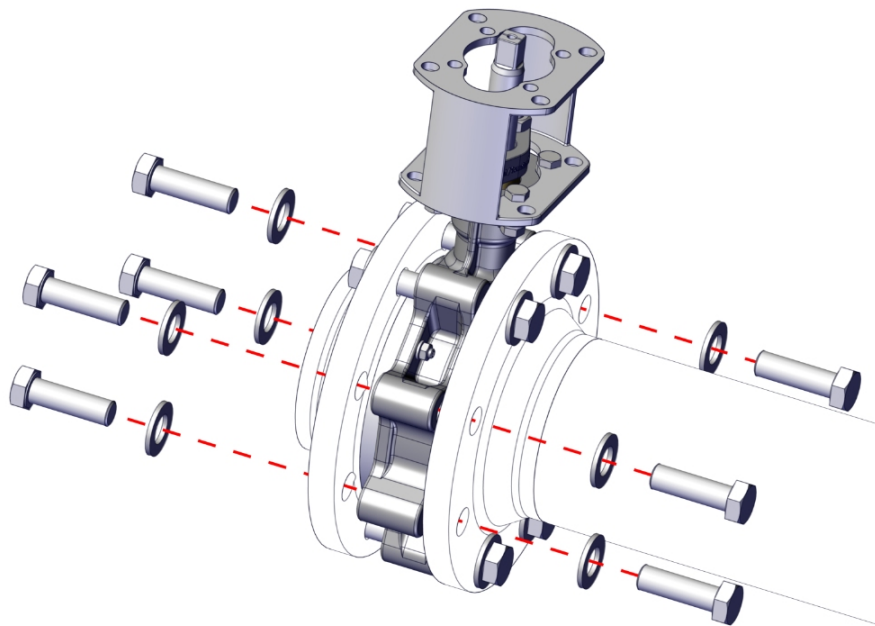
图 9: 用螺栓拧紧法兰连接罩
