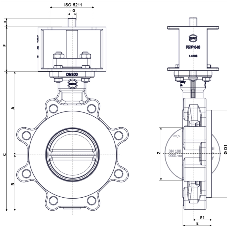
图 3: HP114-HF 主要尺寸
