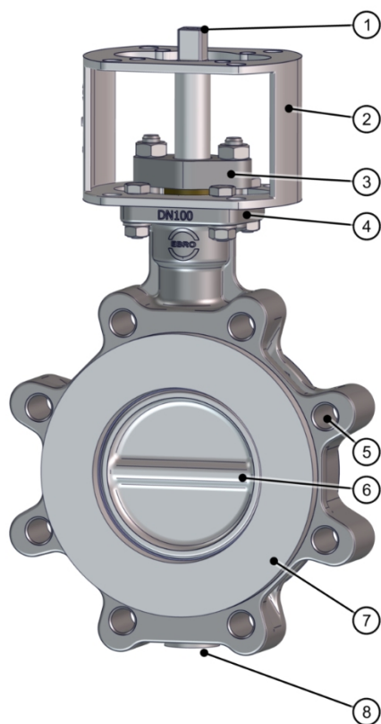
图 2: 组件
