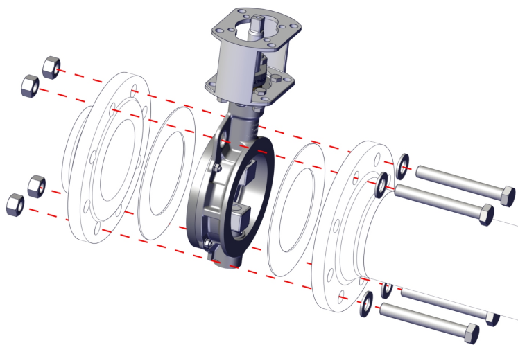
图 8: 定位中间法兰罩
