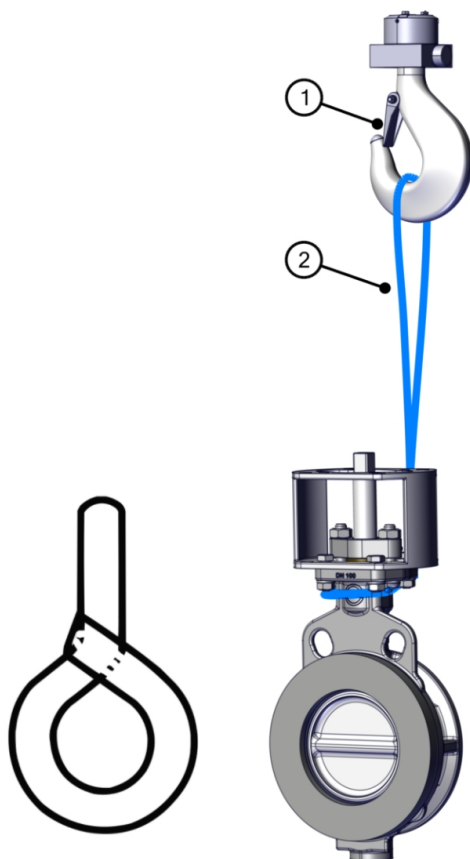
图 6: 起吊中间法兰罩
