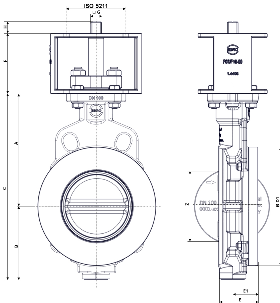
图 3: HP111-HF 主要尺寸
