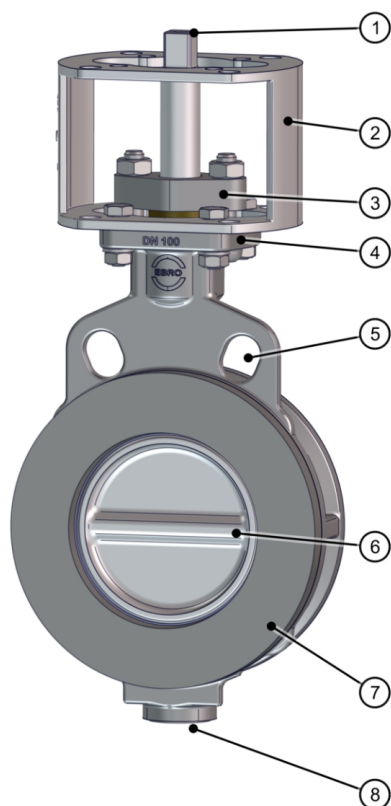
图 2: 组件
