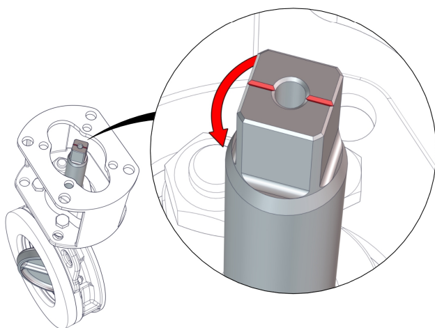
图 14: 操纵方向
