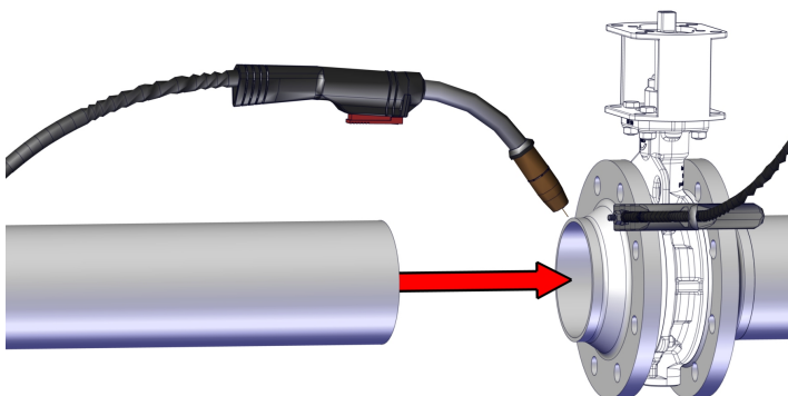
图 10: 将管道与法兰焊接在一起
