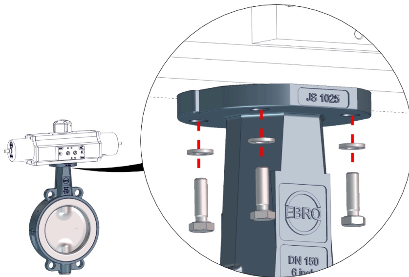
图 7: Prinzip Komponenten montieren
