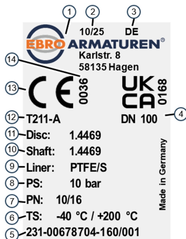
图 1: 铭牌示例
