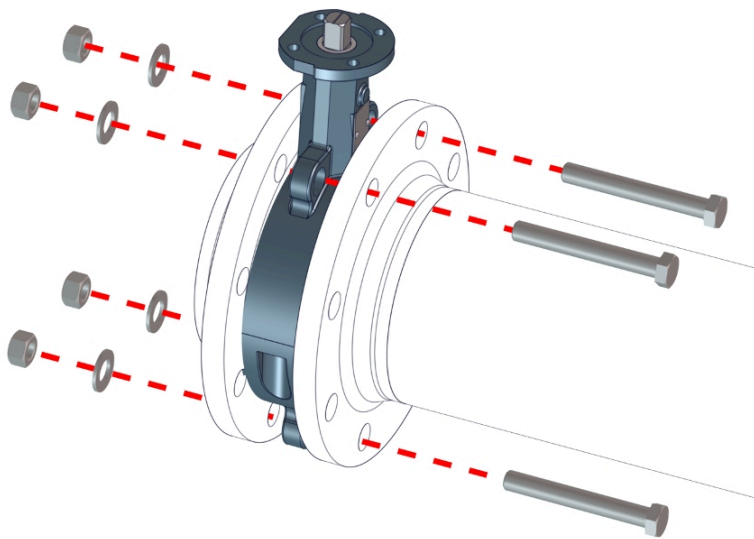
图 8: Zwischenflanschklappe positionieren
