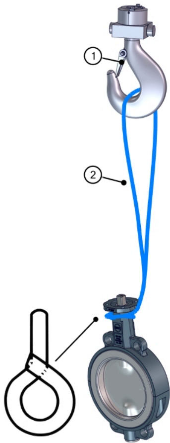
图 6: Zwischenflanschklappe kranen
