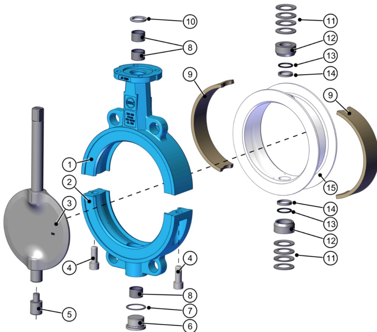
图 16: Stückliste T211-A ab DN40
