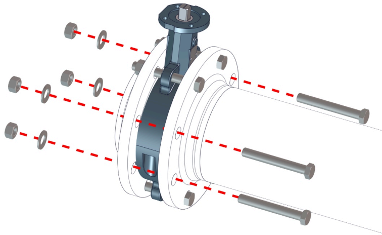
图 9: Zwischenflanschklappe verschrauben
