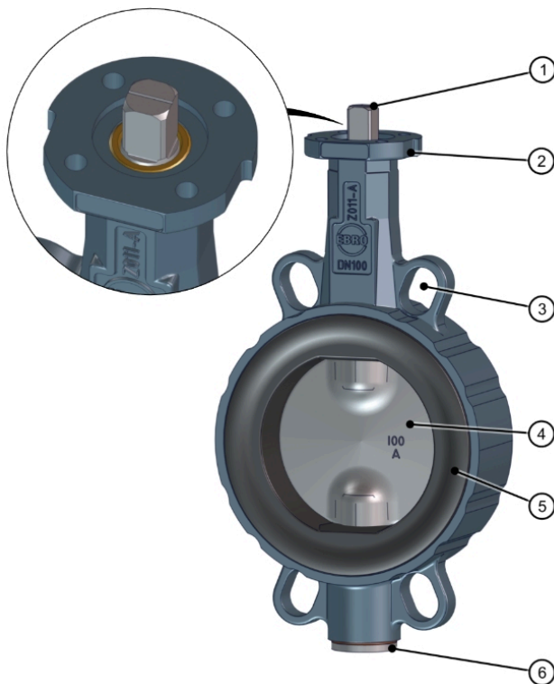
图 2: 组件
