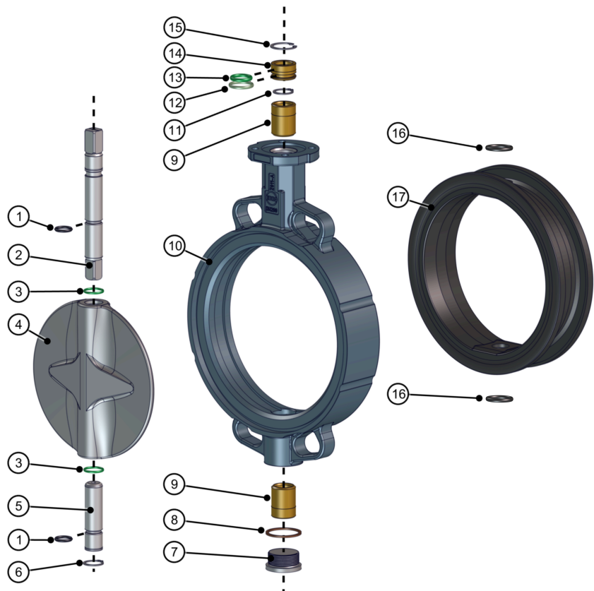
图 19: 2 轴 TS 蝶板零件清单
