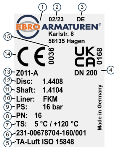
图 1: 铭牌示例
