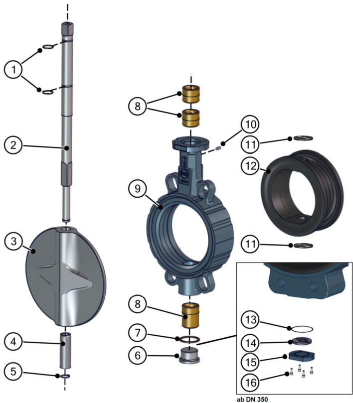
图 16: TS 轴Z011-A零件清单
