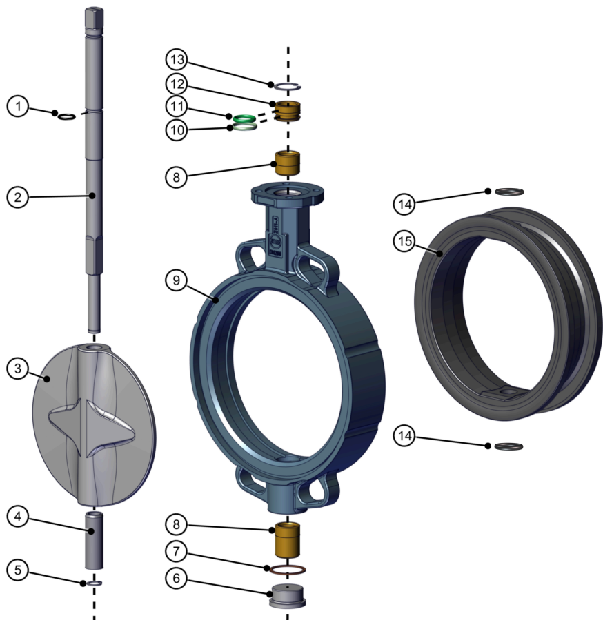
图 18: 1 轴 TS 蝶板零件清单
