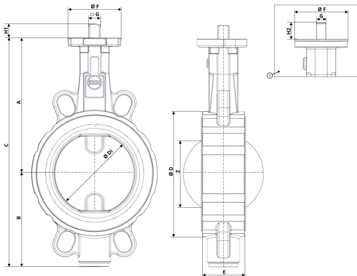
图 3: Z011-A 主要尺寸
