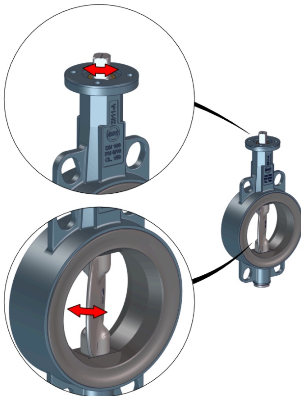
图 4: 可移动零件
