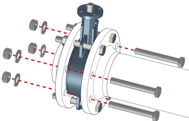
图 9: 用螺栓拧紧中间法兰罩
