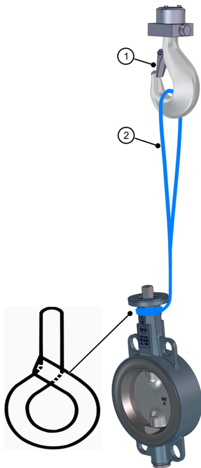
图 6: 起吊中间法兰罩
