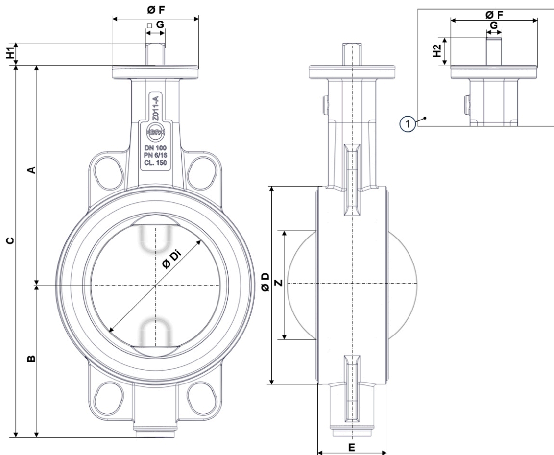
图 3: Z011-AS 主要尺寸
