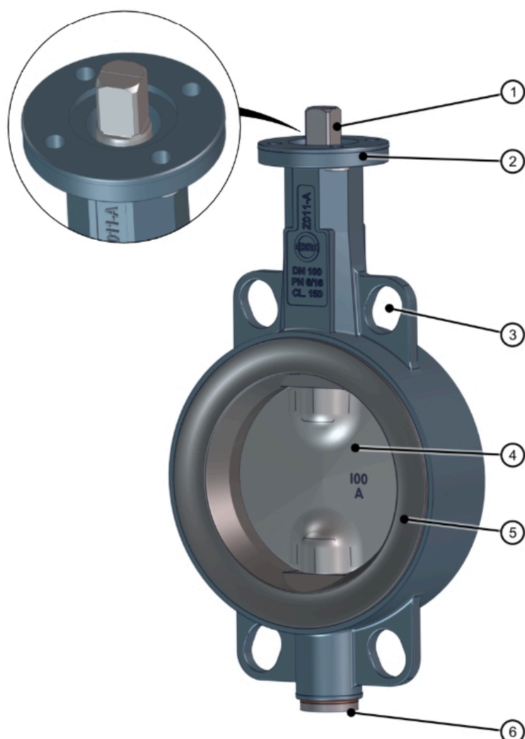
图 2: 组件
