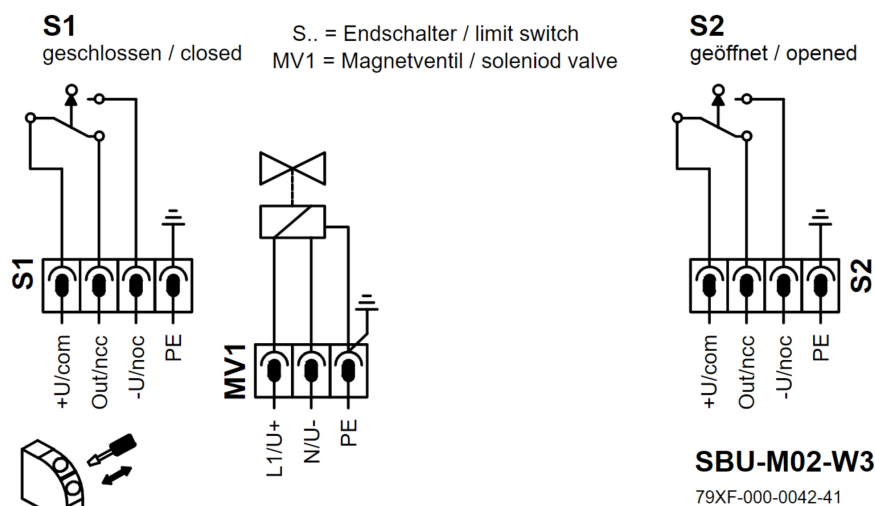
图 7: SBU Basic 电路图
