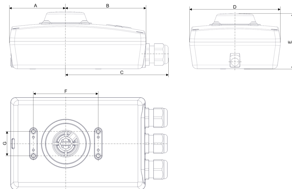
图 4: 尺寸
