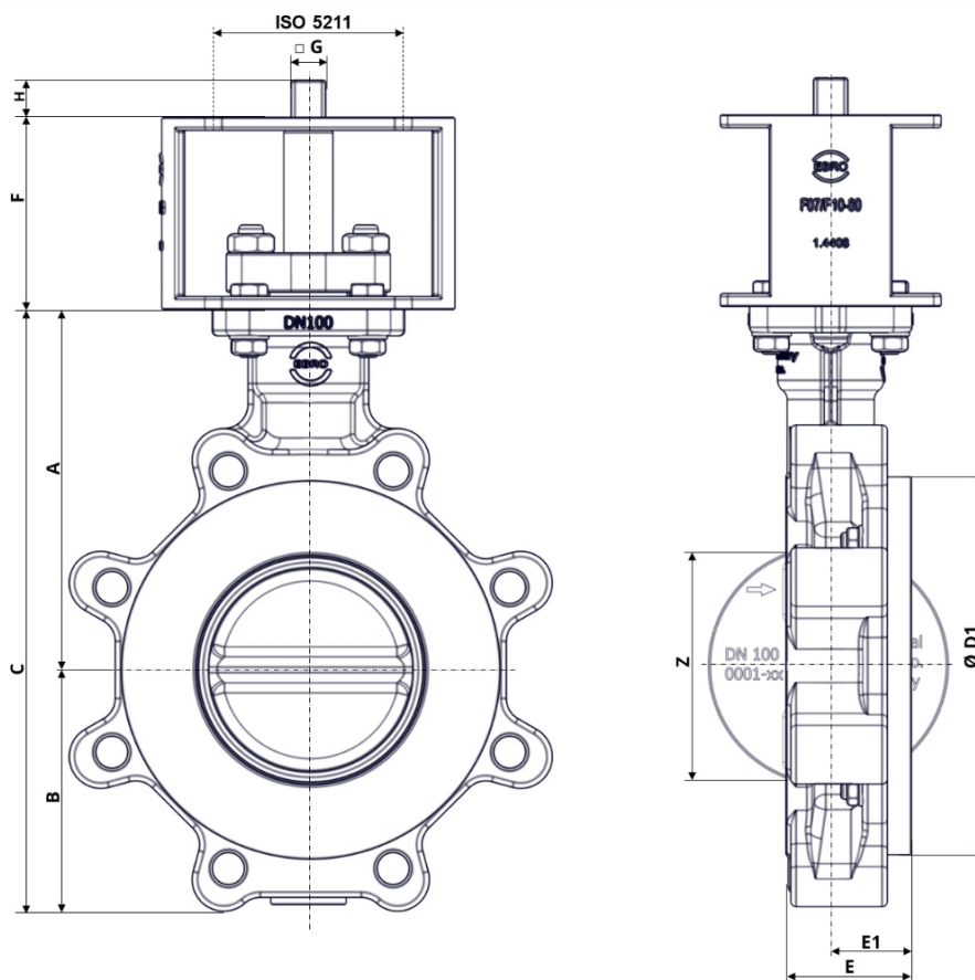
Фиг. 3: Основни размери HP114-HF
