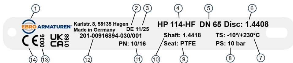
Фиг. 1: Пример типова табелка
