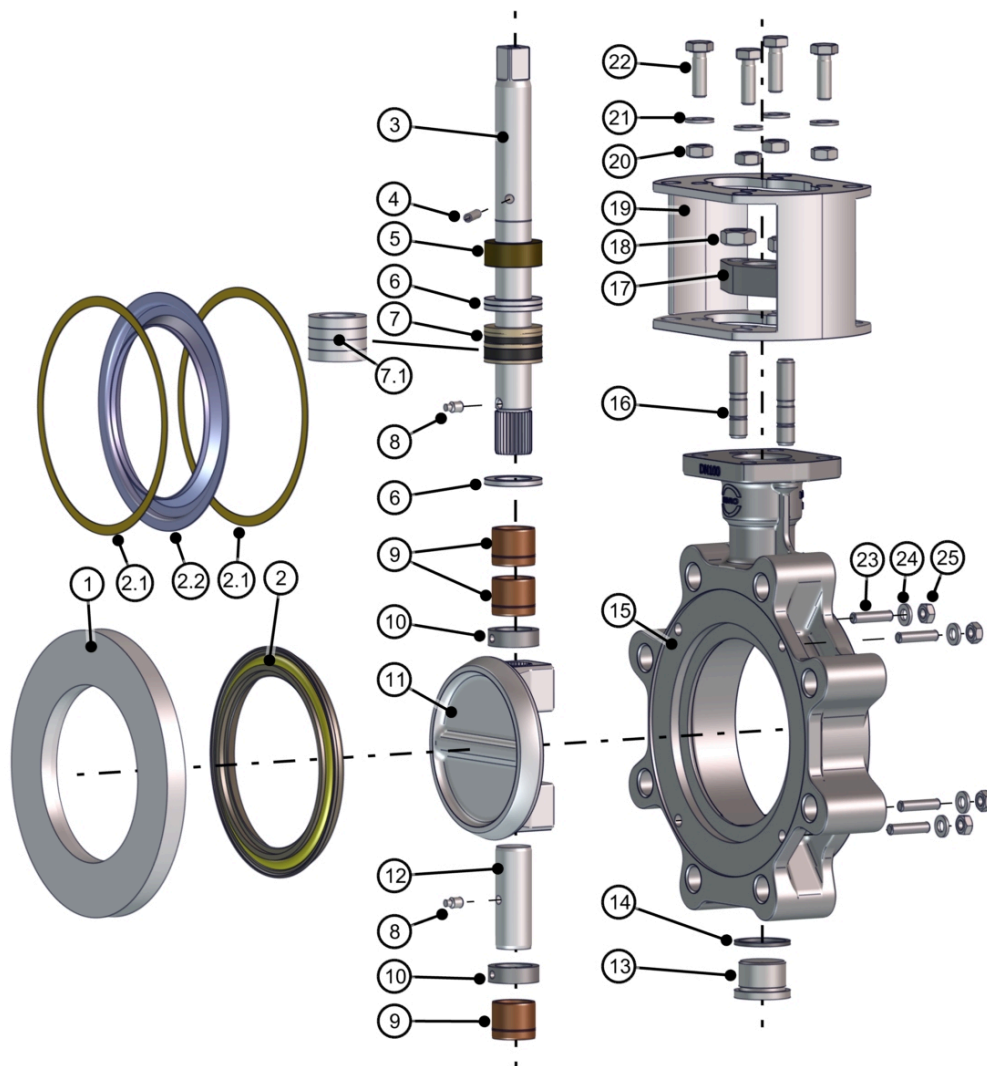
Фиг. 15: Спецификация HP114-HF
