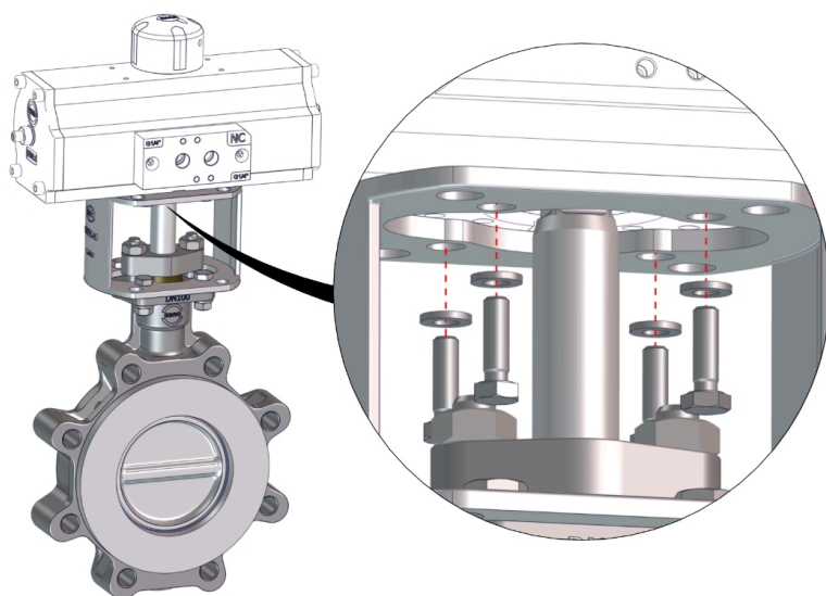
Фиг. 7: Принцип на монтиране на компоненти
