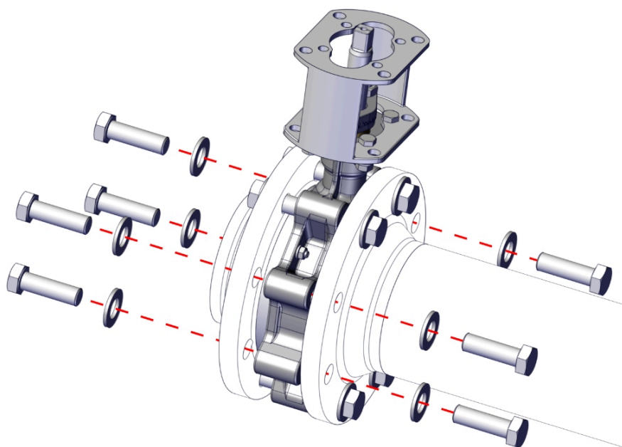
Фиг. 9: Завинтване на фланцовата клапа
