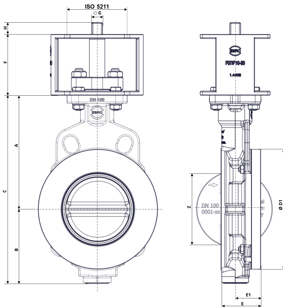
Фиг. 3: Основни размери HP111-HF
