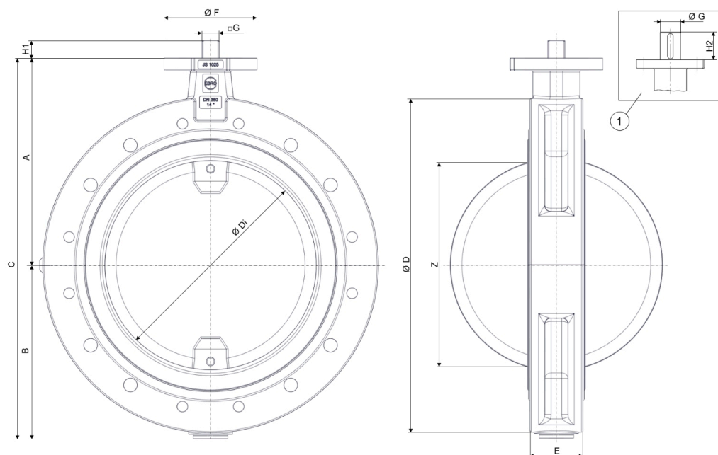
Фиг. 3: Основни размери T212-A
