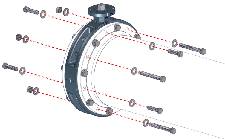
Фиг. 9: Завинтване на двойна фланцова клапа
