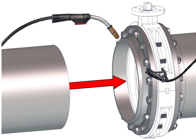
Фиг. 10: Заваряване на тръба с фланец
