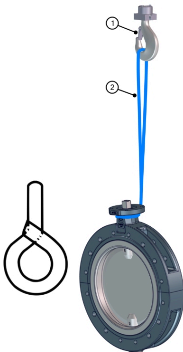
Фиг. 6: Повдигане с кран на двойна фланцова клапа
