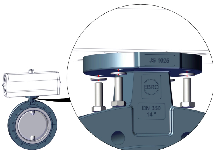
Фиг. 7: Принцип на монтиране на компоненти
