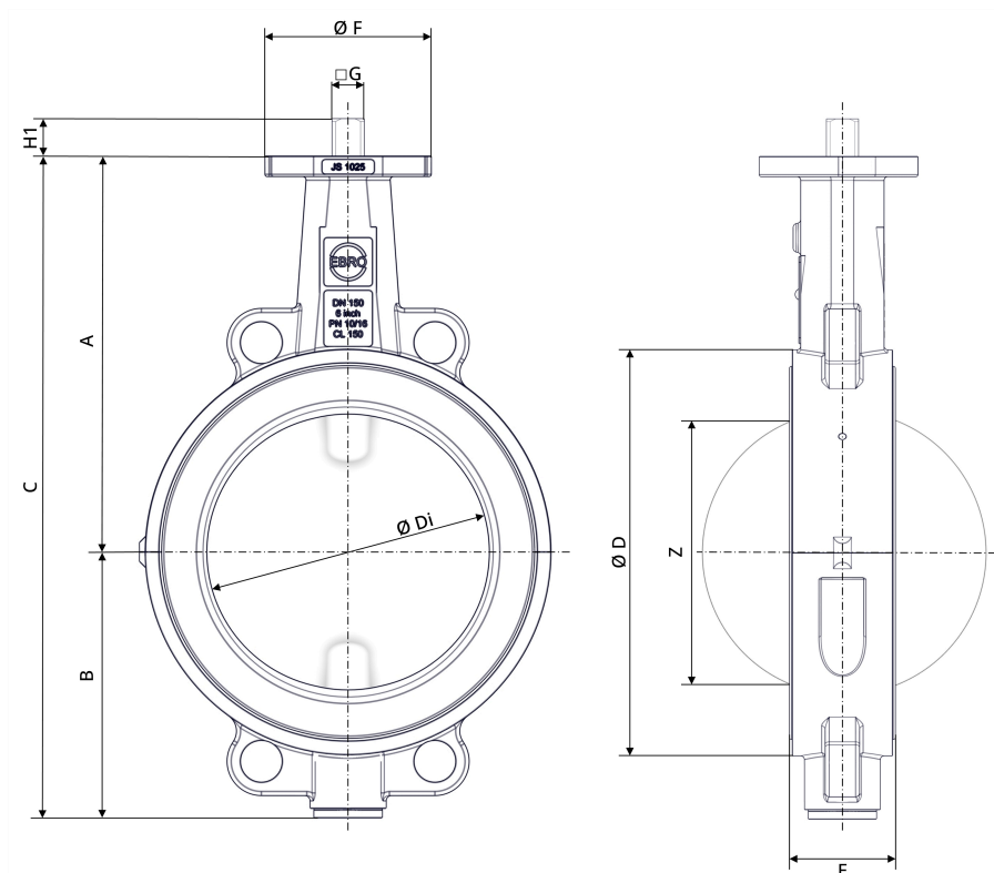
Фиг. 3: Основни размери T211-A
