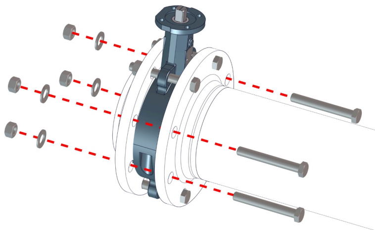
Фиг. 9: Zwischenflanschklappe verschrauben
