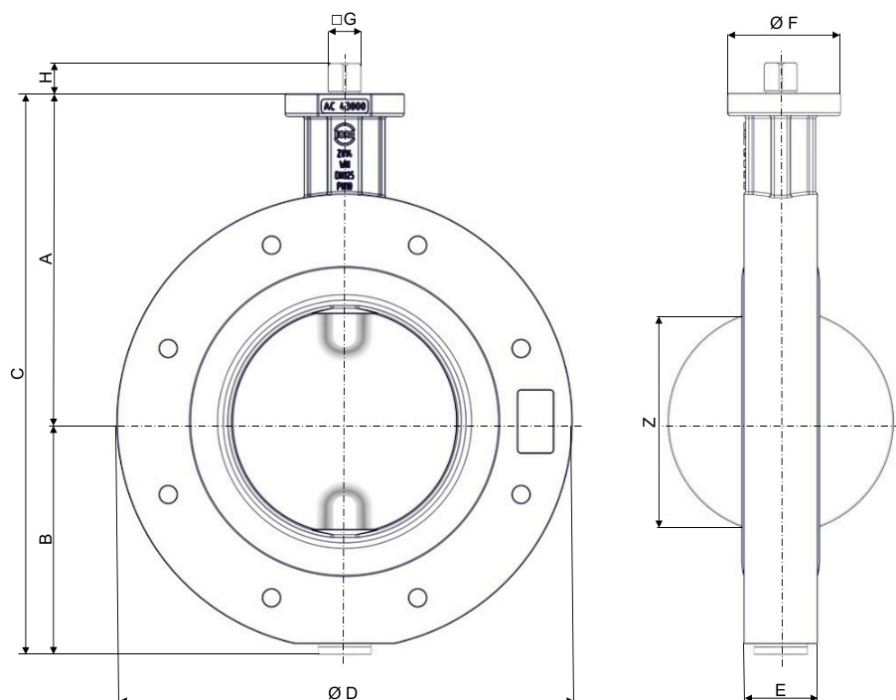
Фиг. 3: Основни размери Z014-WN
