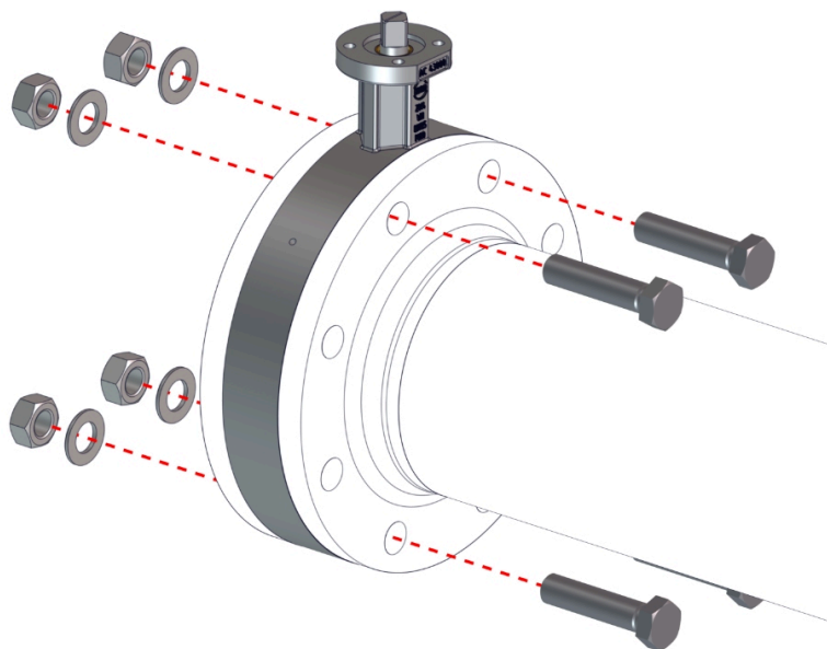
Фиг. 8: Позициониране на пълна фланцова клапа
