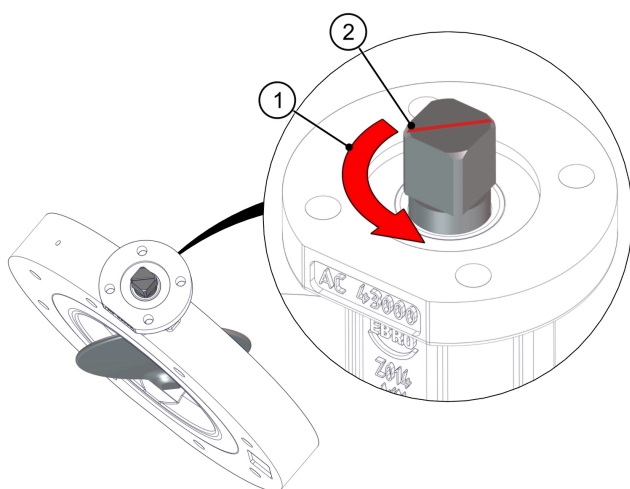
Фиг. 14: Посока на задействане
