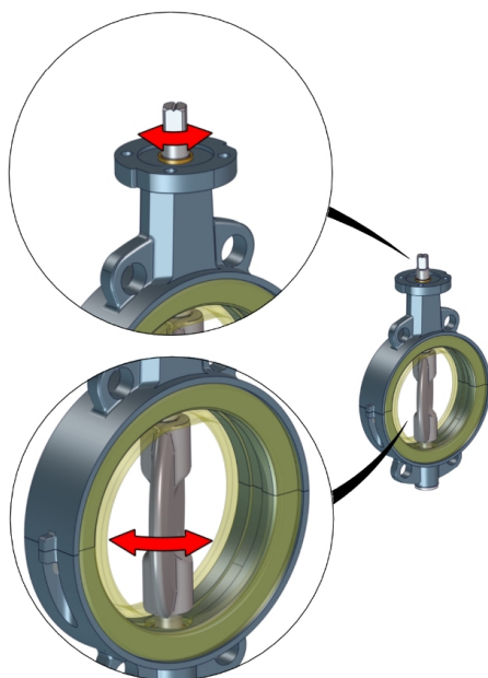
Фиг. 4: Подвижни части
