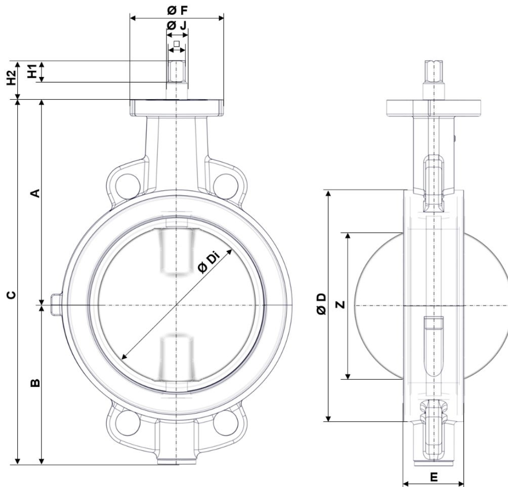
Фиг. 3: Основни размери Z011-GMX
