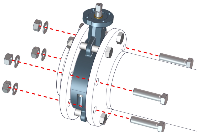
Фиг. 9: Завинтване на междинната фланцова клапа
