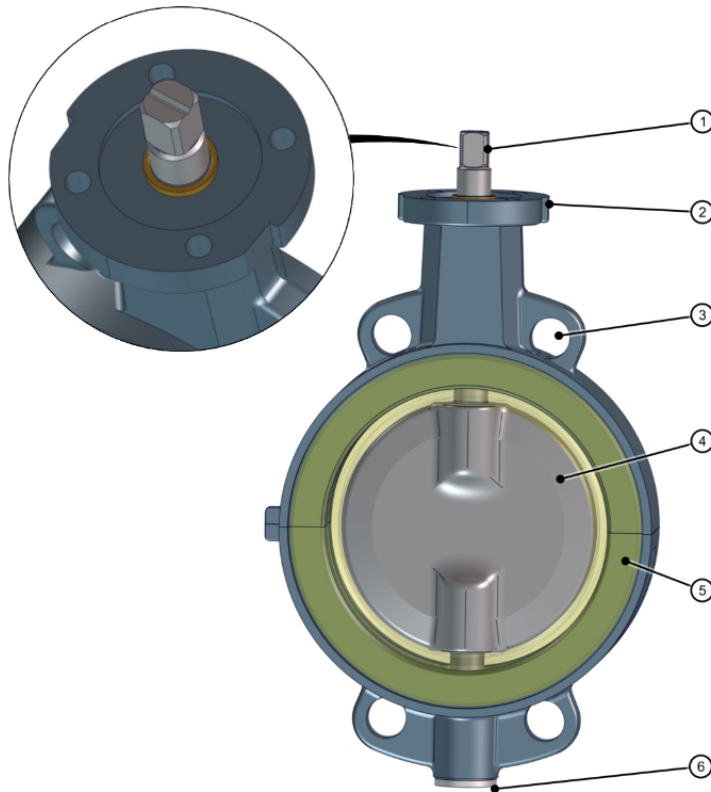
Фиг. 2: Компоненти
