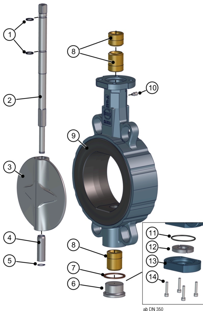
Фиг. 16: Спецификация Z011-B TS-вал
