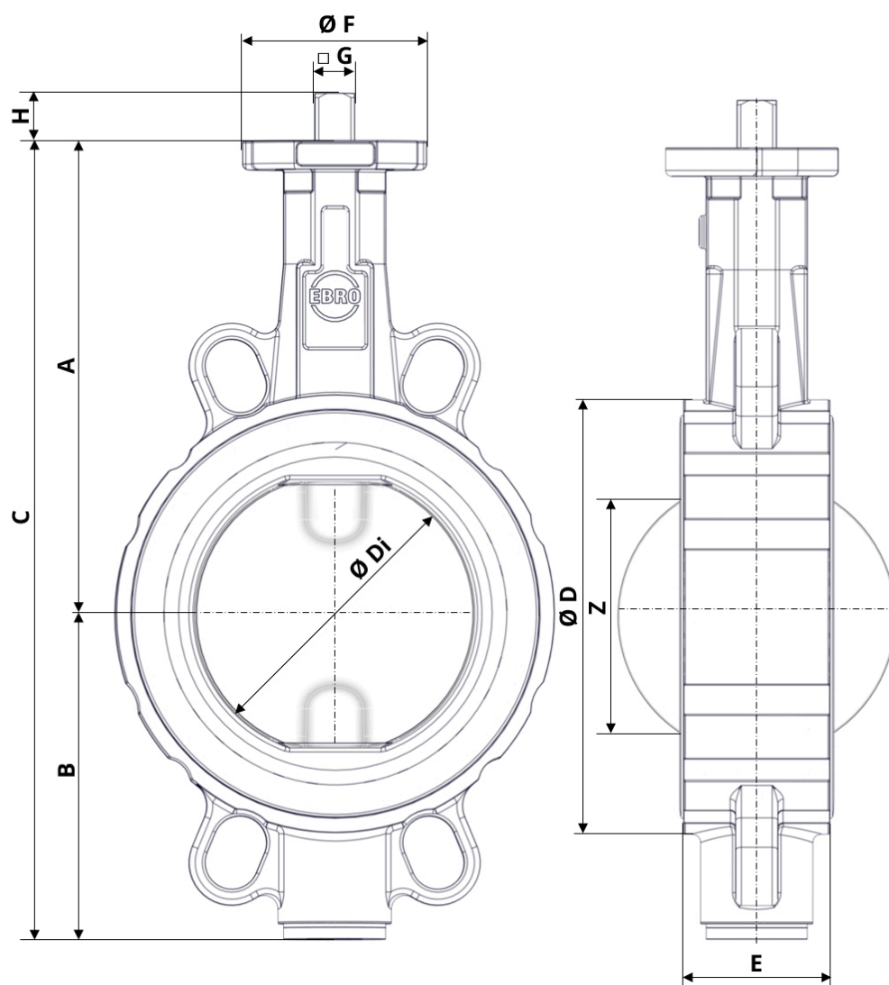
Фиг. 3: Основни размери Z011-B
