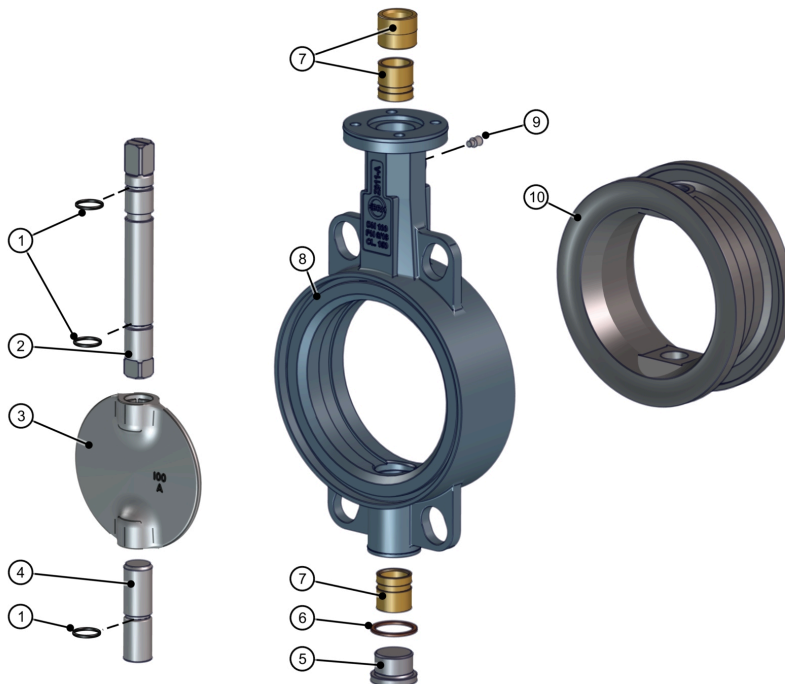
Фиг. 15: Спецификация Z011-AS
