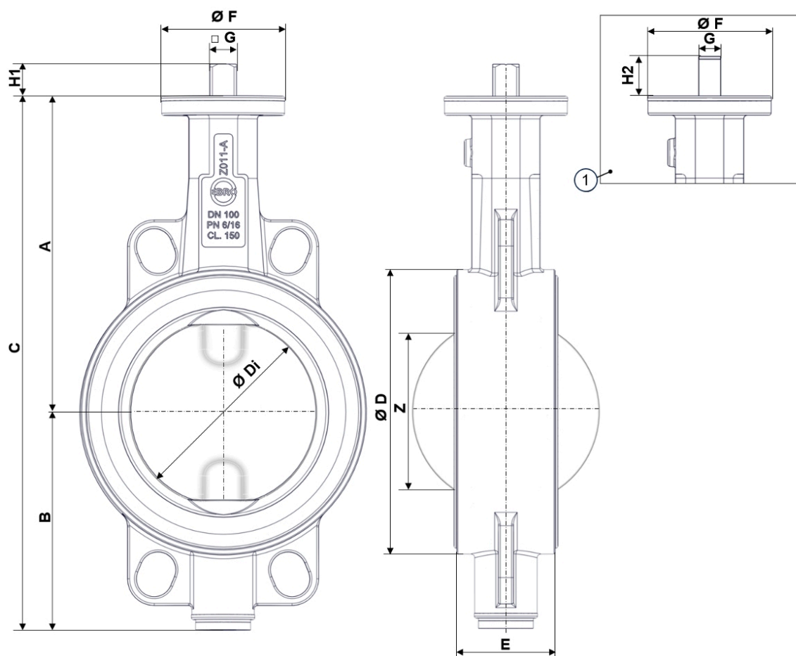
Фиг. 3: Основни размери Z011-AS
