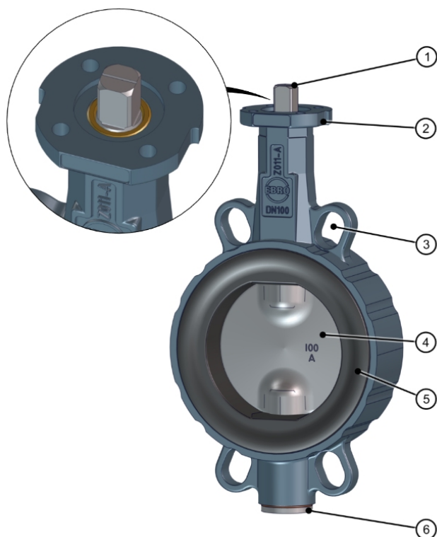
Фиг. 2: Компоненти
