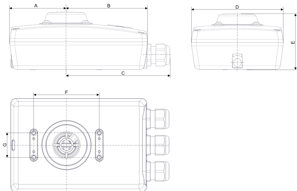
Фиг. 4: Размери
