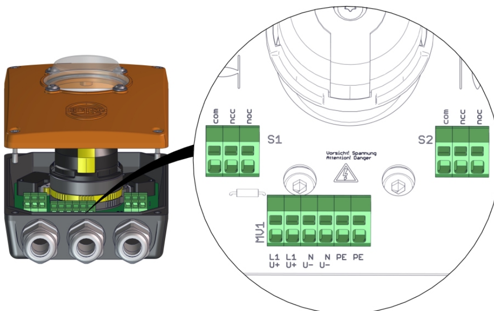
Фиг. 6: Щекерна лисна за SBU-Basic
