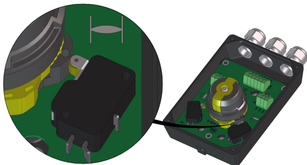
Фиг. 9: Настройка на ексцентрика „ЗАТВОРЕНО“
