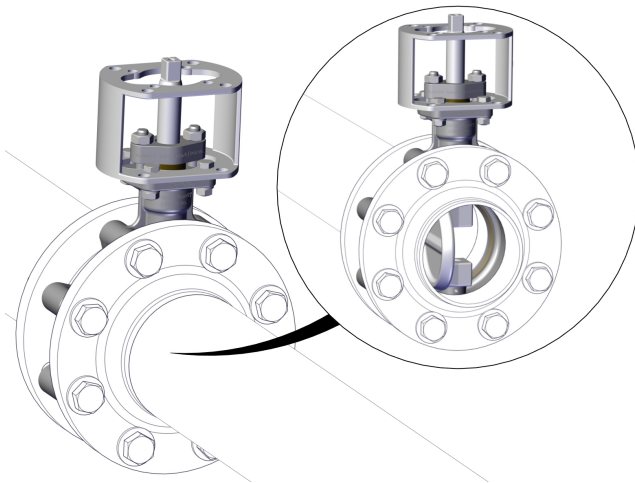
Abb. 13: Rohr spülen
