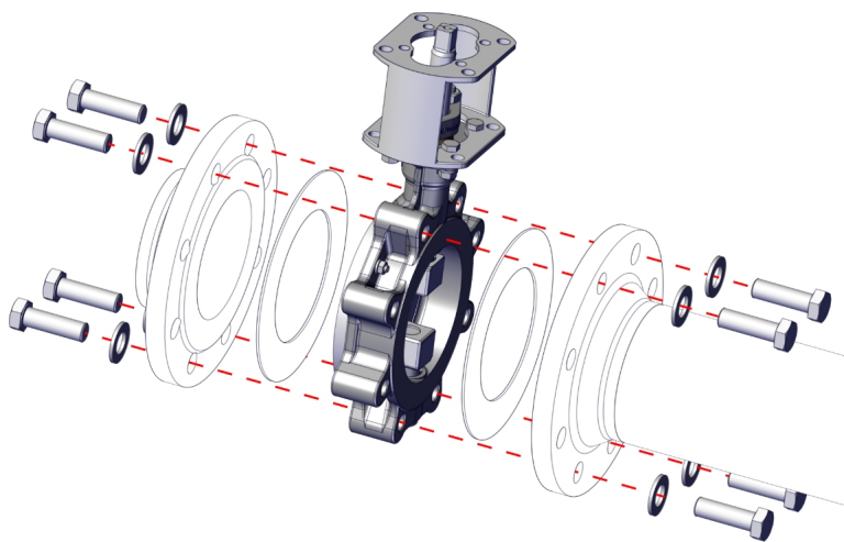
Abb. 8: Anflanschklappe positionieren
