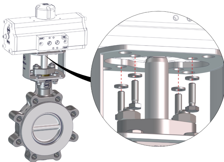
Abb. 7: Prinzip Komponenten montieren
