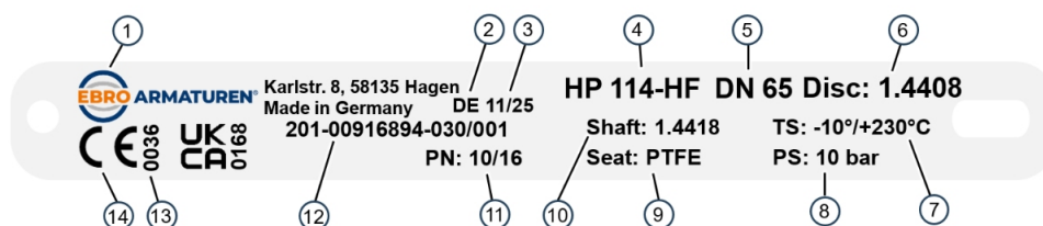
Abb. 1: Beispiel-Typenschild
