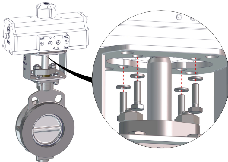
Abb. 7: Prinzip Komponenten montieren
