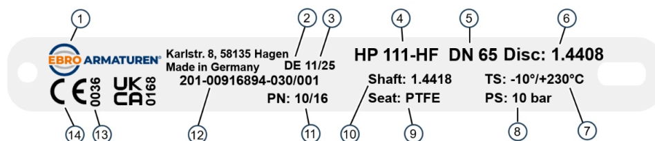
Abb. 1: Beispiel-Typenschild
