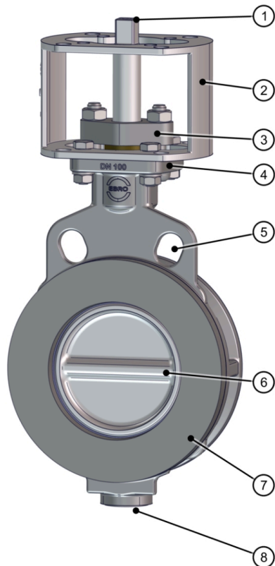
Abb. 2: Komponenten
