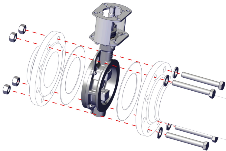
Abb. 8: Zwischenflanschklappe positionieren
