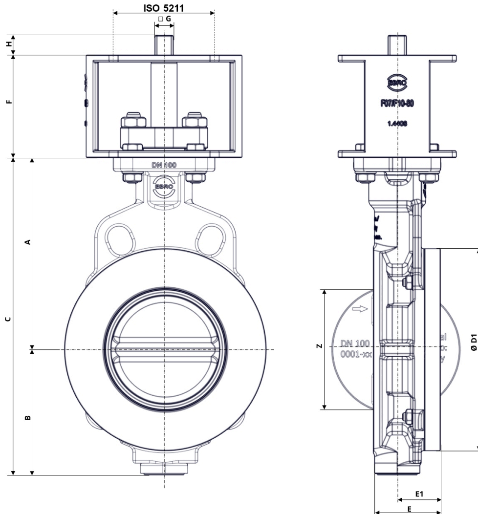
Abb. 3: Hauptabmessungen HP111-HF
