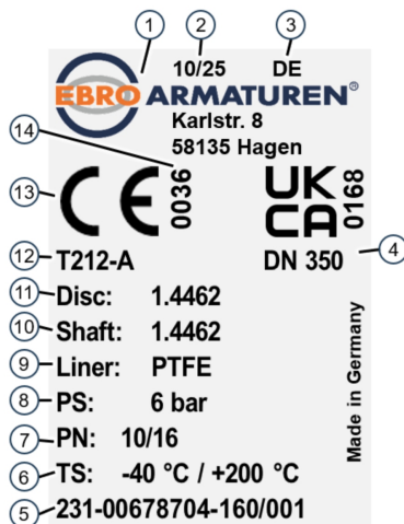
Abb. 1: Beispiel Typenschild
