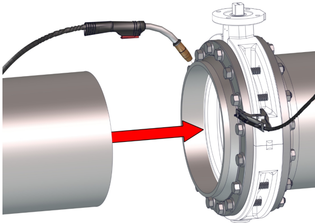
Abb. 10: Rohr mit Flansch verschweißen
