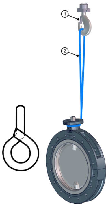
Abb. 6: Doppelflanschklappe kranen
