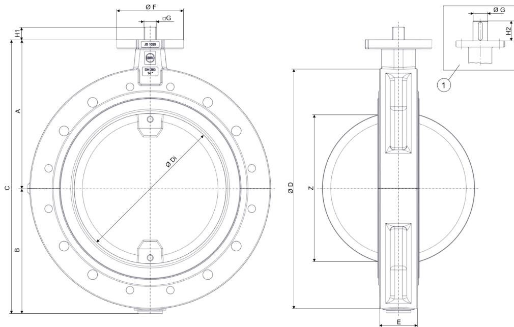
Abb. 3: Hauptabmessungen T212-A
