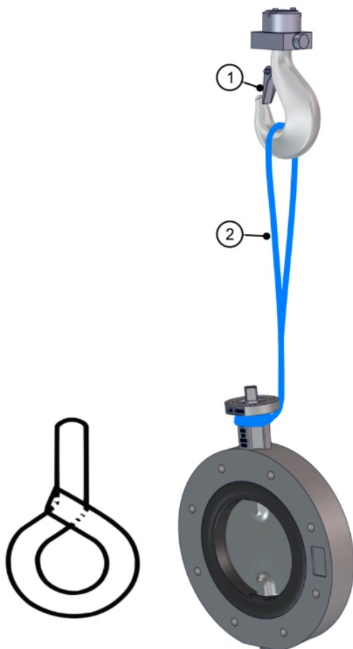
Abb. 6: Vollflanschklappe kranen
