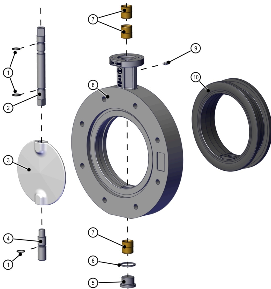
Abb. 15: Stückliste Z014-WN
