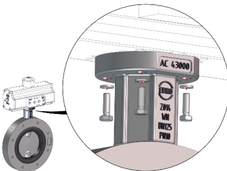
Abb. 7: Prinzip Komponenten montieren
