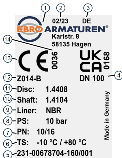
Abb. 1: Beispiel-Typenschild
