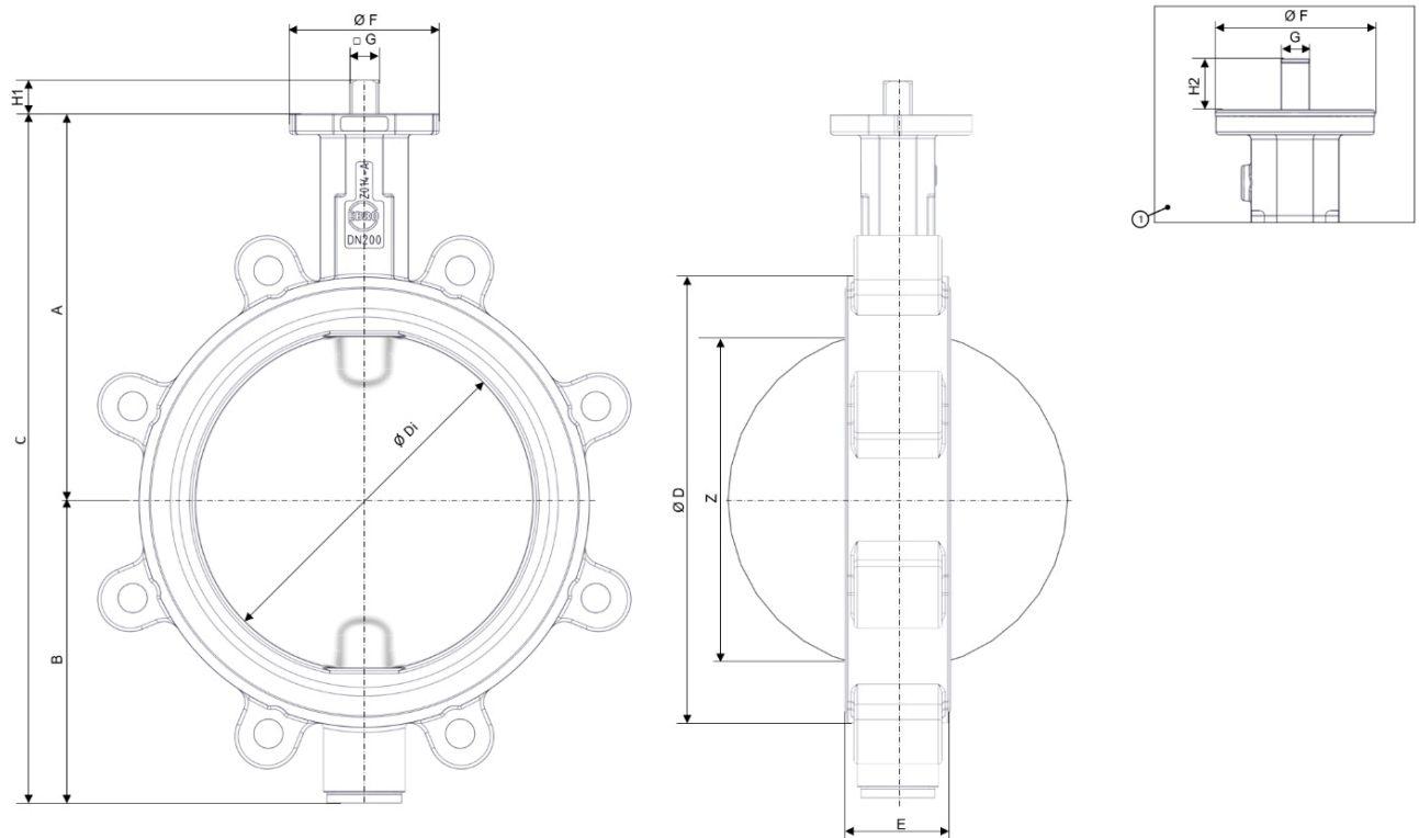
Abb. 3: Hauptabmessungen Z014-B
