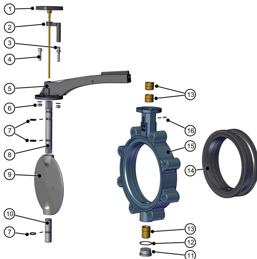
Abb. 16: Stückliste Z014-A THERM
