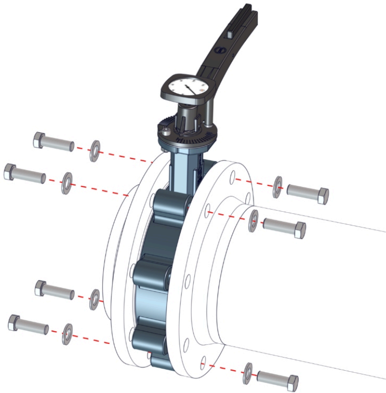
Abb. 8: Anflanschklappe positionieren
