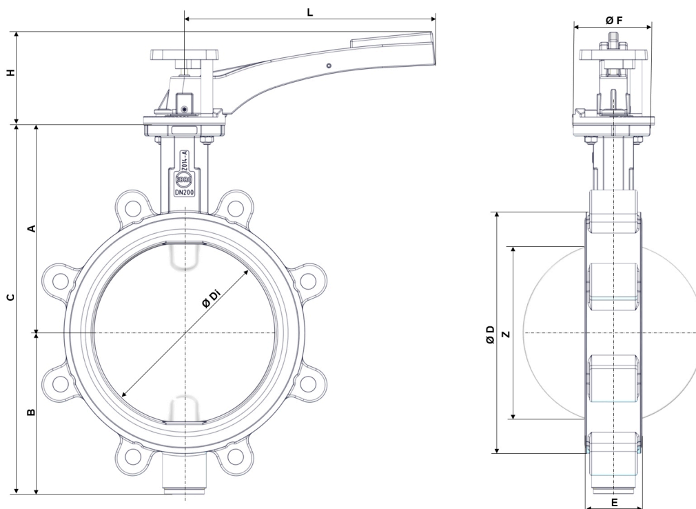
Abb. 3: Hauptabmessungen Z14-A THERM
