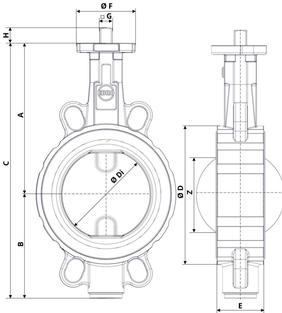
Abb. 3: Hauptabmessungen Z011-B
