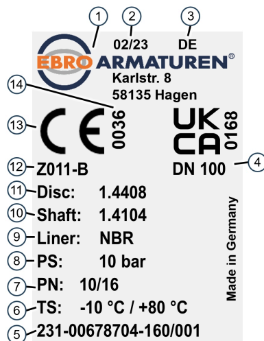
Abb. 1: Beispiel-Typenschild
