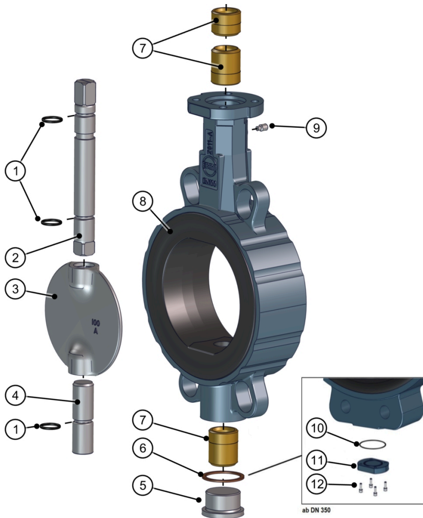
Abb. 15: Stückliste Z011-B geteilte Welle
