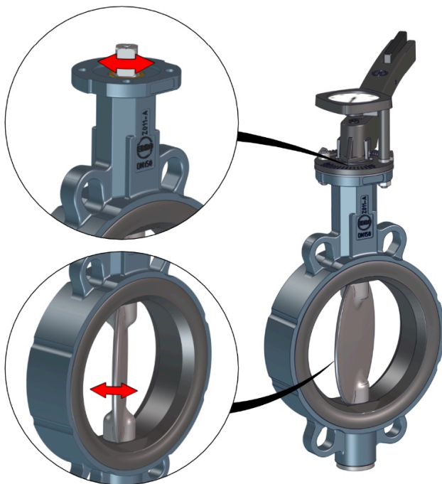
Abb. 4: Bewegliche Teile
