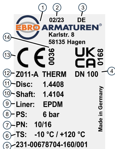
Abb. 1: Beispiel-Typenschild
