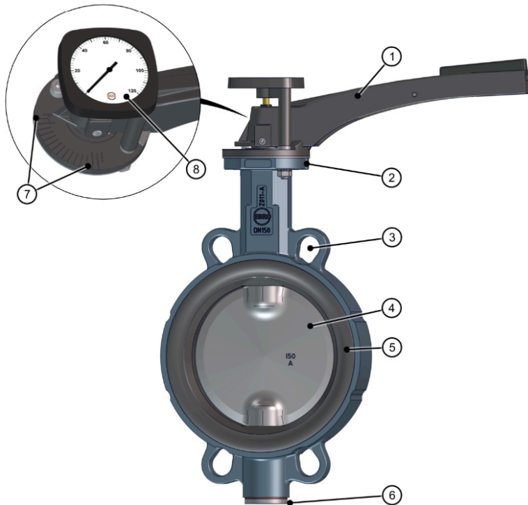
Abb. 2: Komponenten
