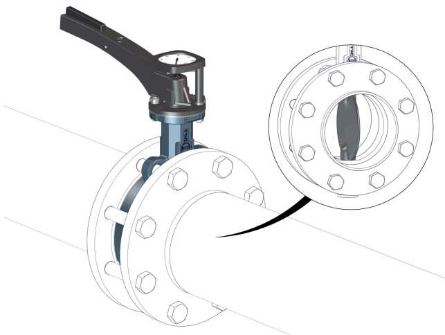
Abb. 13: Rohr spülen
