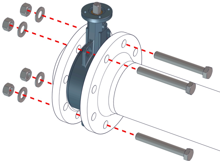
Abb. 8: Zwischenflanschklappe positionieren
