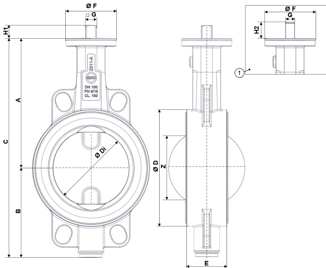
Abb. 3: Hauptabmessungen Z011-AS
