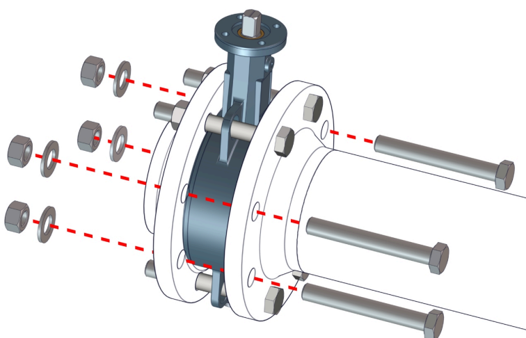
Abb. 9: Zwischenflanschklappe verschrauben
