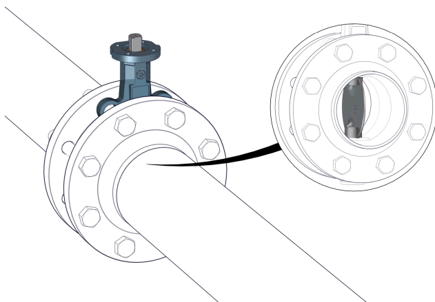
Abb. 13: Rohr spülen
