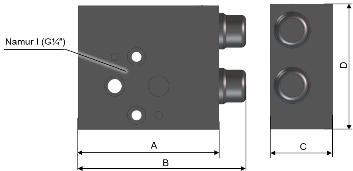
节流模块尺寸表
