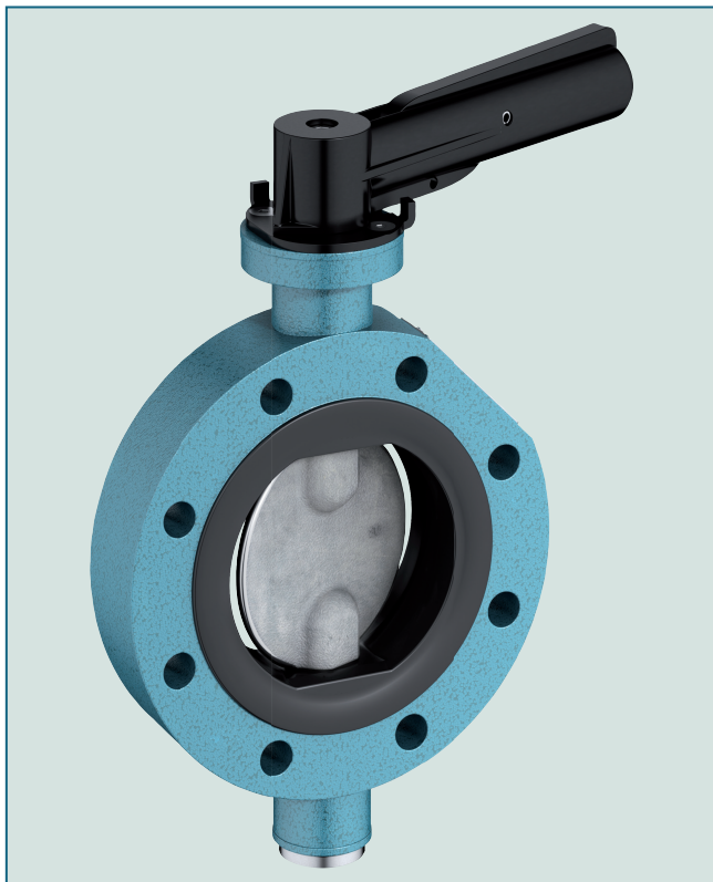
Tankwagenabsperrklappe Typ TW 100 mit NBR-Manschette.
