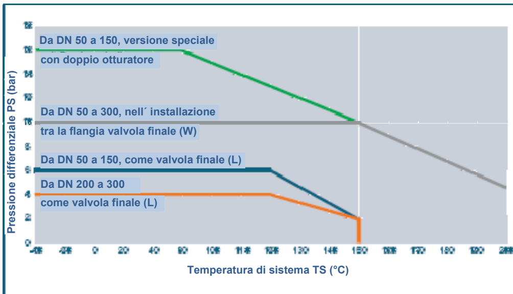
Campo inserto a vuoto nel montaggio tra la flangia: fino a 1 mbar, con -10 C° a 160 C°
